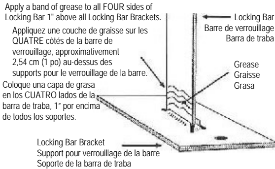
Fig. 6 Internal Locking Bar and Guide Bracket Barre interne de verrouillage et support de guidage Barra interna de traba y soporte de guía
