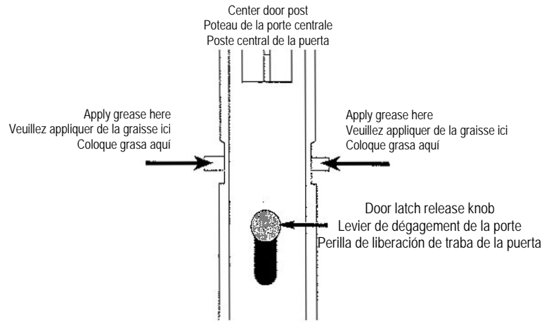
Fig. 8 Lock Pins Goupille d'arrêt Clavijas de traba
